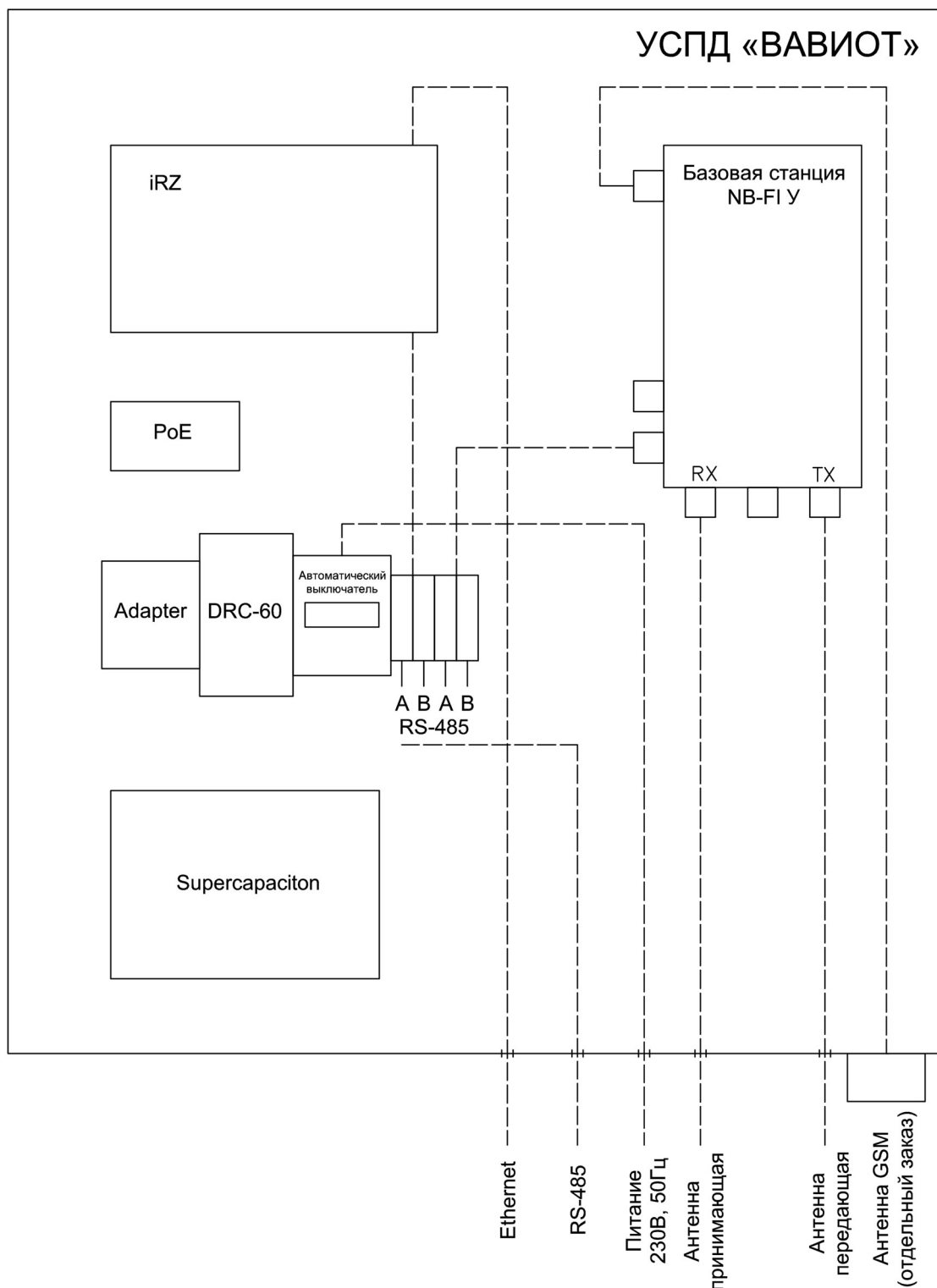
Рисунок Б1 – Схема подключения УСПД
