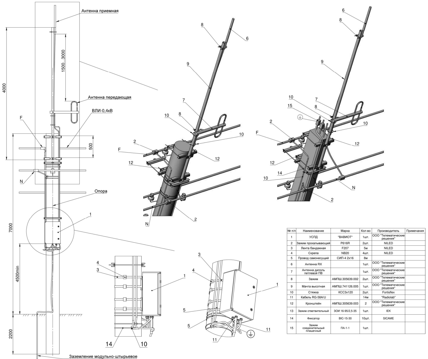
Рисунок В1 – Техническое решение по установке УСПД (установка на опору ЛЭП 0,4 кВ)
